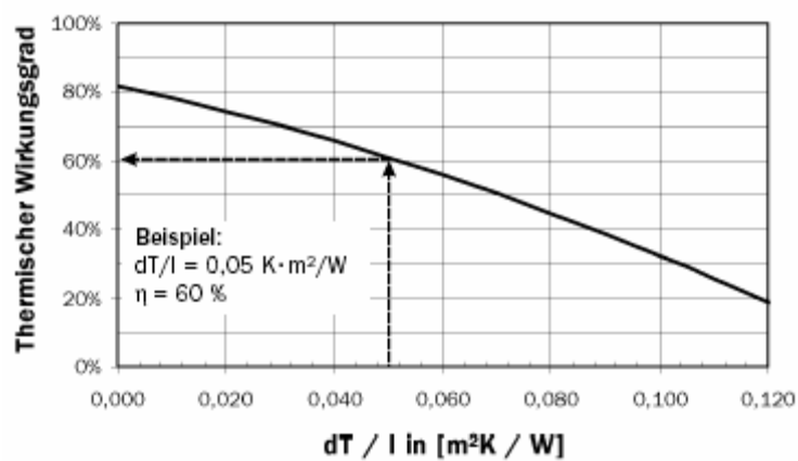
Wirkungsgrad-Kennlinie SolvisCala
