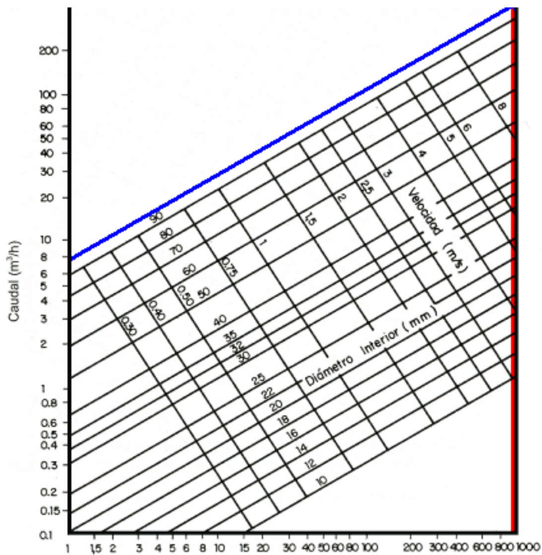
Pérdida por rozamiento (mm c.a. por m) para tubería de cobre
