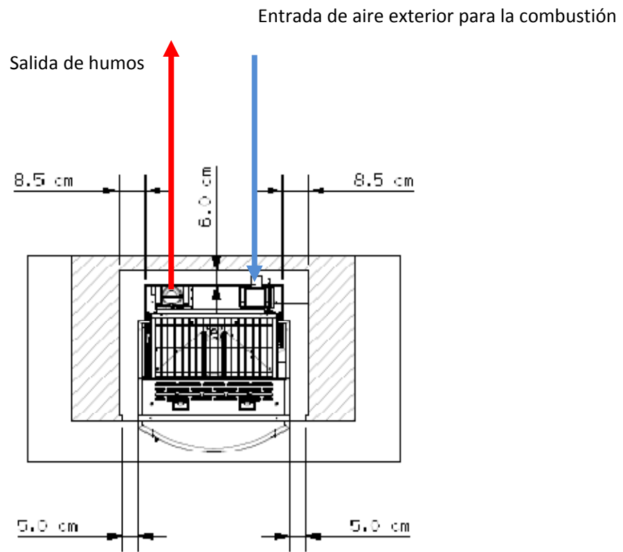
Vista en planta de equipo confort maxi
