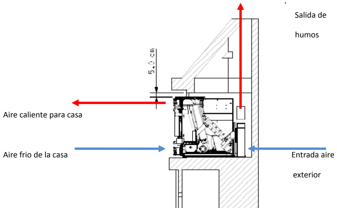
Corte en sección
