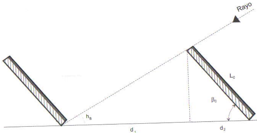
Figura 1.16. Sombreado entre colectores.
