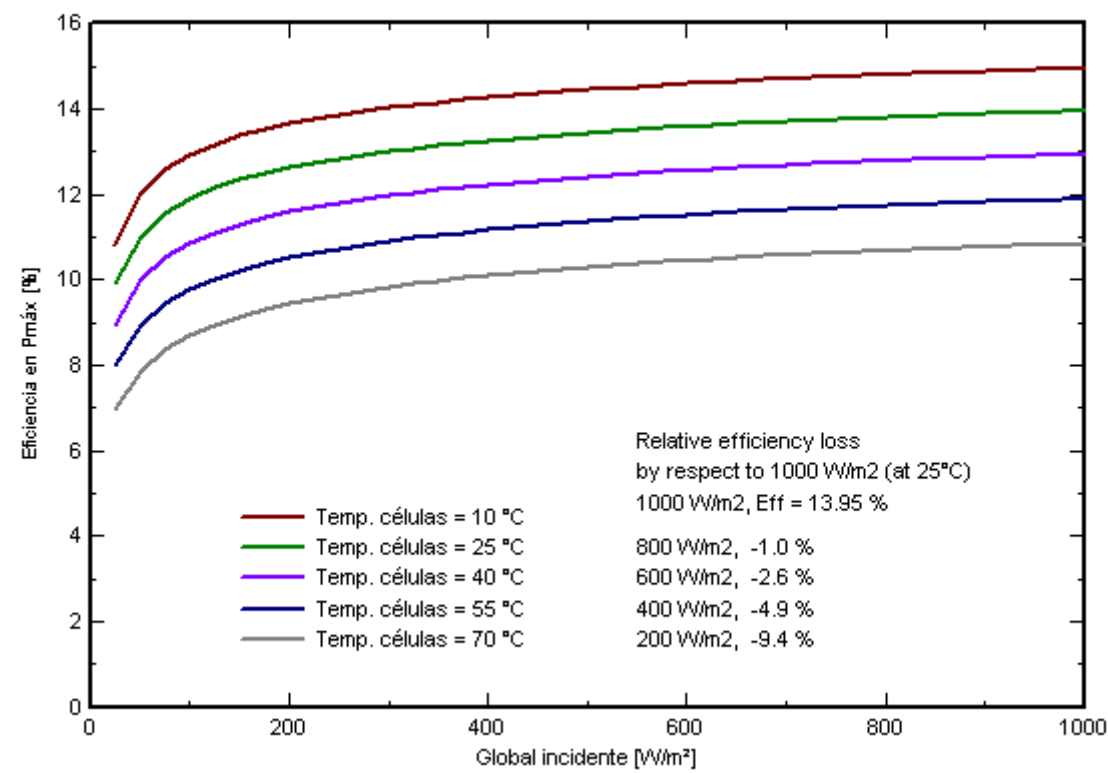
Módulo FV: Suntech, STP 270-24/Vb
