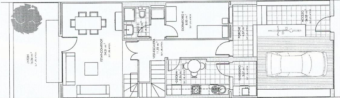
Planta baja
